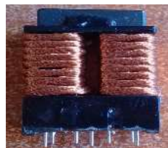
谐振电感 UU25 35mm*20mm*50mm 3KW 15A 220V
